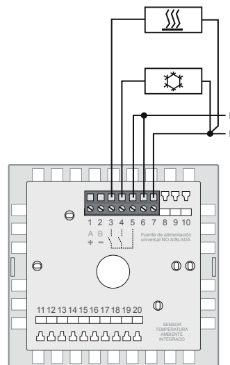
ESQUEMA 2: Regulación frío y calor
