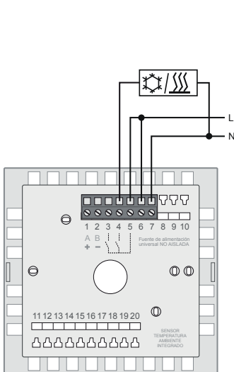
ESQUEMA 3: Regulación frío/calor
