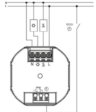
Esquema de conexión UTE 4100-Rw
