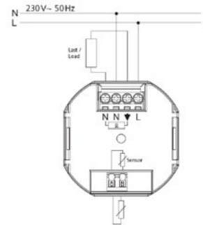
Esquema de conexión UTE 4800-R
