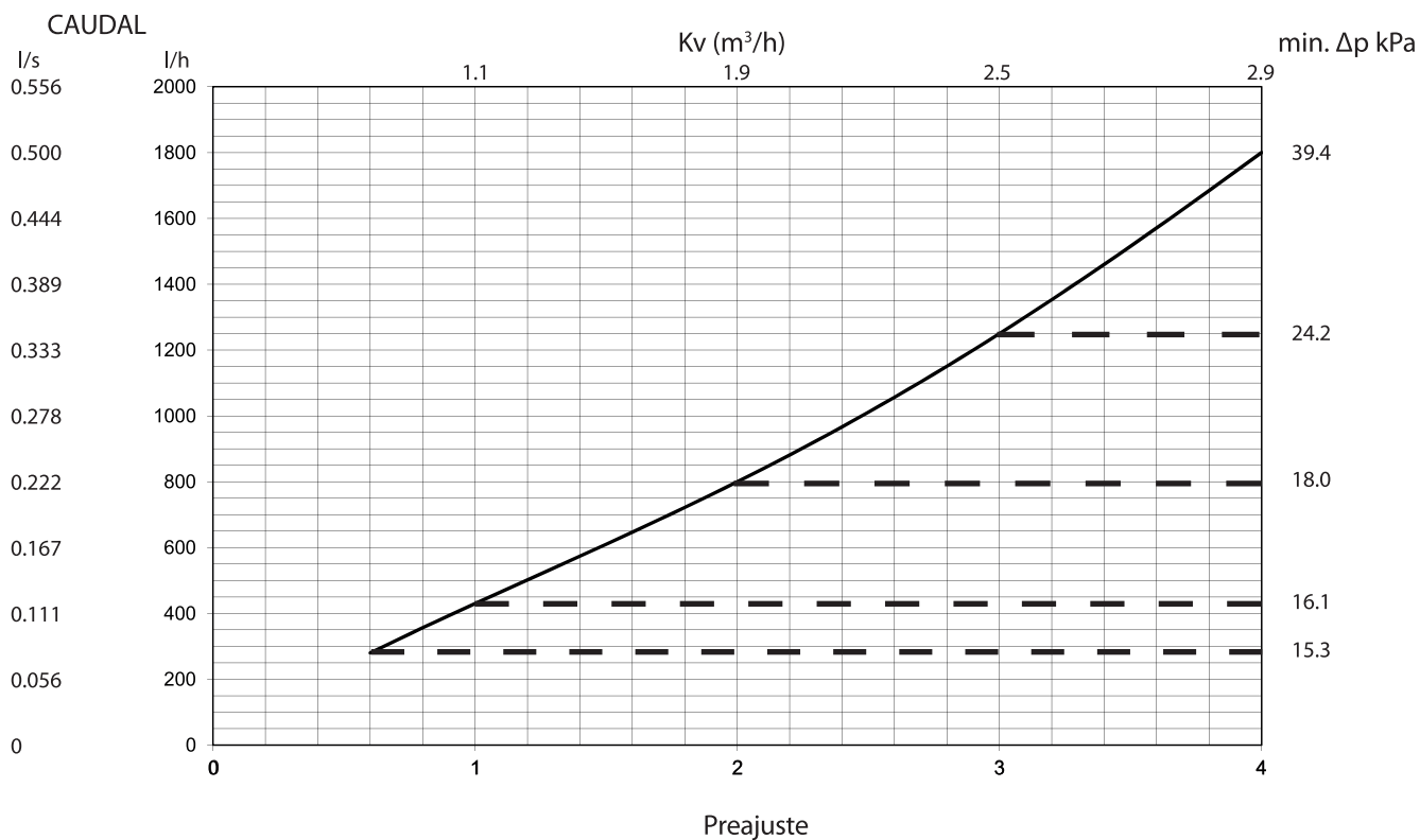
Gráfica de caudales Frese OPTIMA Compact caudal bajo 5,5mm DN25
