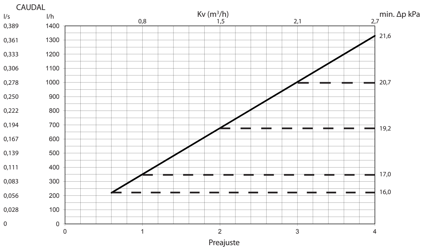
Gráfica de caudales Frese OPTIMA Compact caudal alto 5,0mm DN15/20
