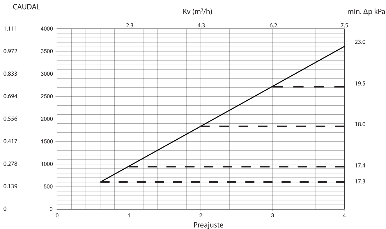
Gráfica de caudales Frese OPTIMA Compact 5,5mm DN32
