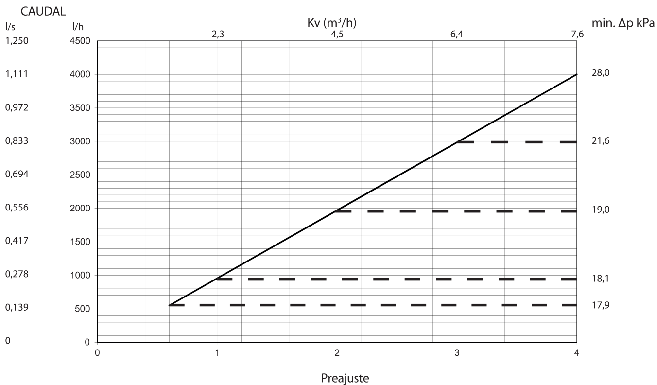
Gráfica de caudales Frese OPTIMA Compact 5,5mm DN32
