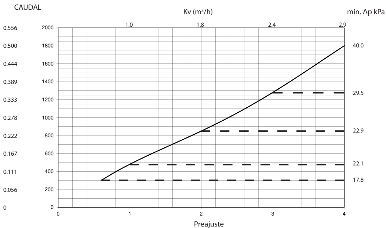
Gráfica de caudales Frese OPTIMA Compact caudal bajo 5,5mm DN25
