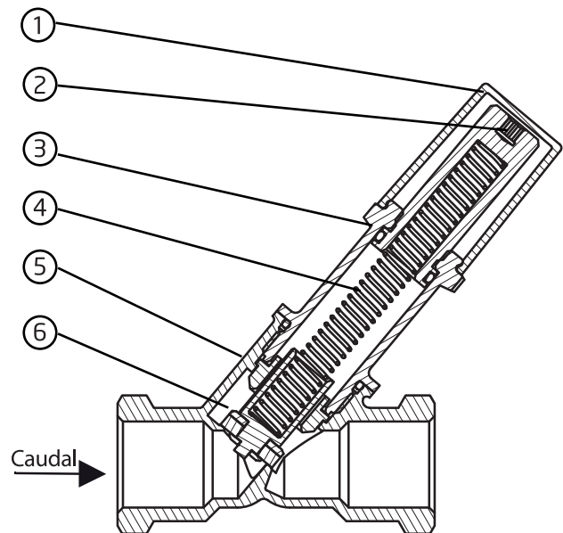
Dibujo de sección transversal Frese DPRV
